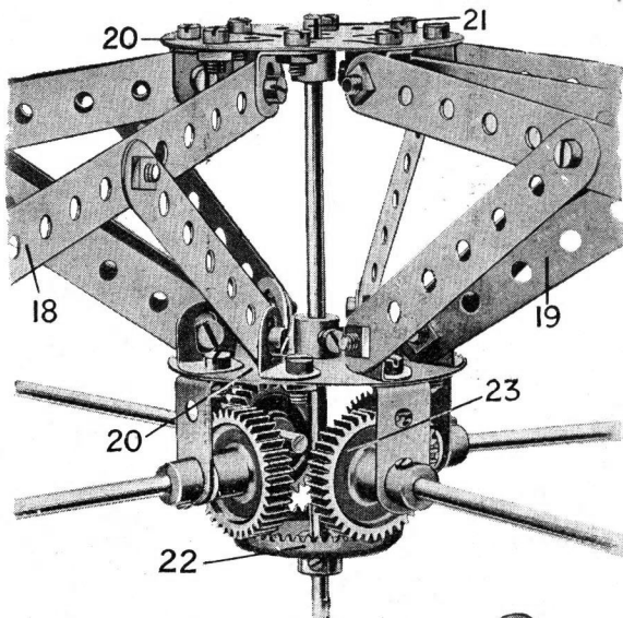
Fig. 6. — Mécanisme supérieur de commande
