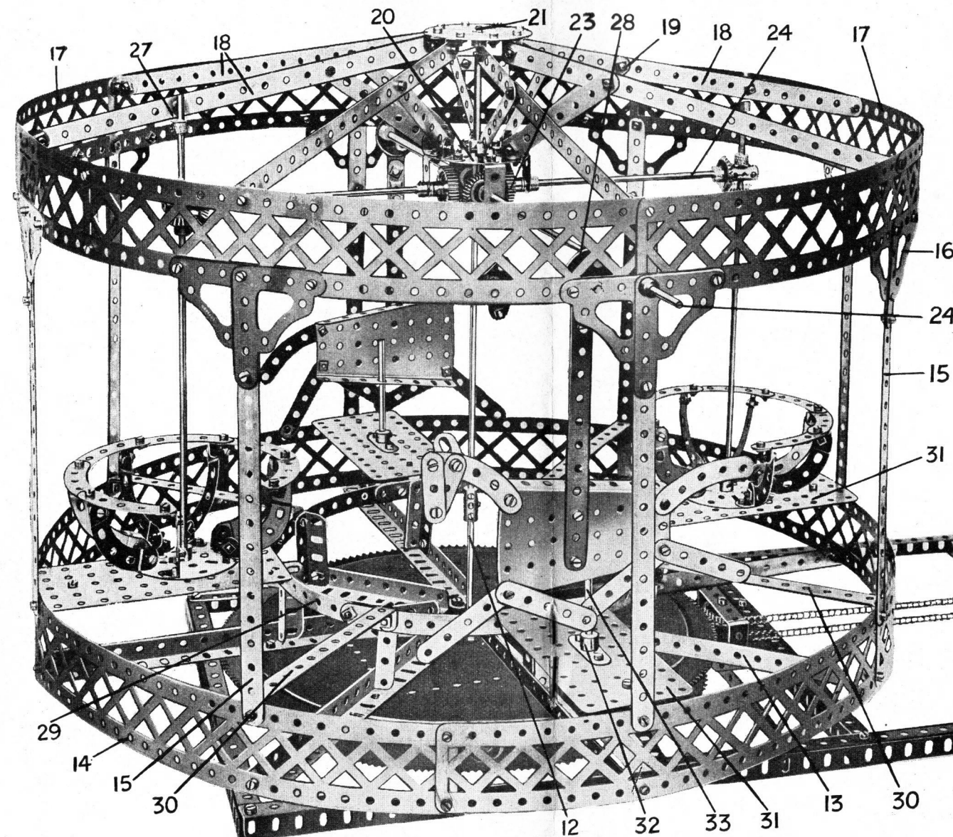
Fig. 1. Vue générale du Manège
