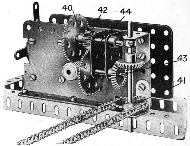
Fig. 3. — Mécanisme monté sur le Moteur électrique
