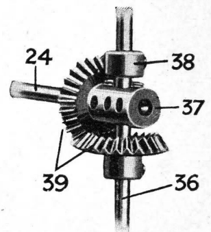
Fig. 4. — Mécanisme commandant les Voitures tournantes
