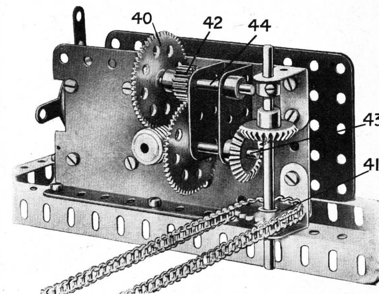
Fig. 3. — Mécanisme monté sur le Moteur électrique
