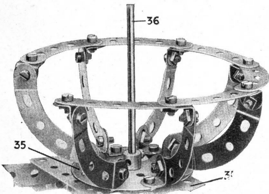
Fig. 2. — Voiture tournante
