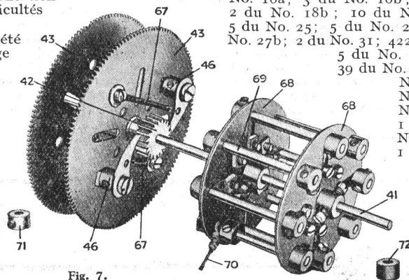
Fig. 7. Le Mécanisme d'Encliquetage.
