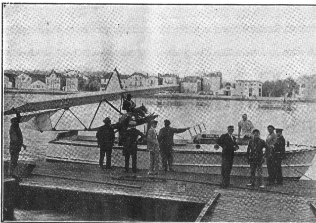
La photographie ci-dessus représente le montage en girouette sur rotule, d'un planeur « Avia ». Ce montage permet à l'élève d'acquiescer tous les réflexes transversaux et longitudinaux dès que le bateau atteint la vitesse nécessaire à la sustentation du planeur. Ce procédé donne une assurance à l'élève et évite tous les accidents du début. Cliché de la Revue « L'Air ».
