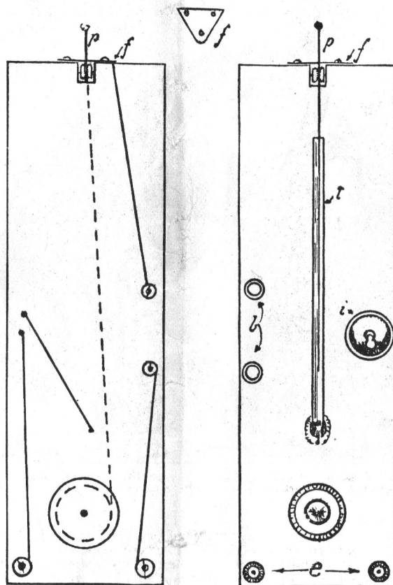
Schéma du rhéostat décrit sur cette page.
