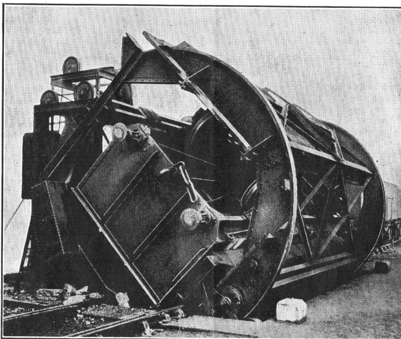
Un Culbuteur de Wagons Rotatif en action. Ce type d'appareil est employé généralement pour le déchargement du charbon aux dépôts de locomotives et aux grandes usines.
