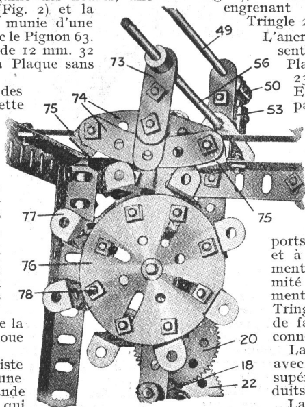
Fig. 4. Le Dispositif d'Échappement.
