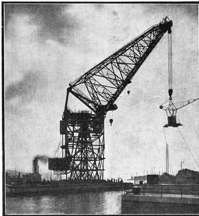
Grue flottante de 150 tonnes.
