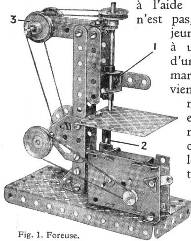
Fig. 1. Foreuse.
