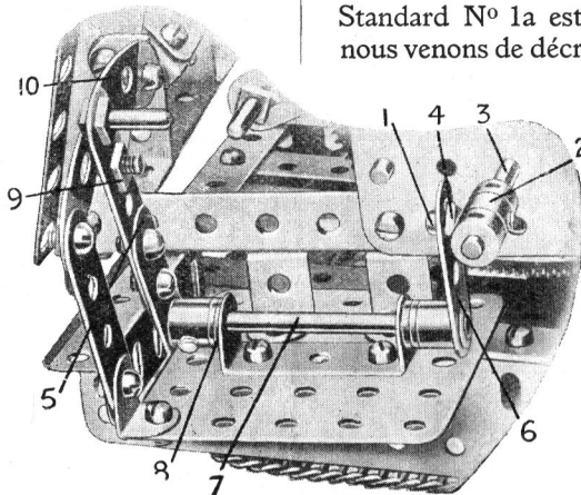
Fig. 1. — Mécanisme à levier, comportant des exemples intéressants de l'emploi des boulons Meccano.
