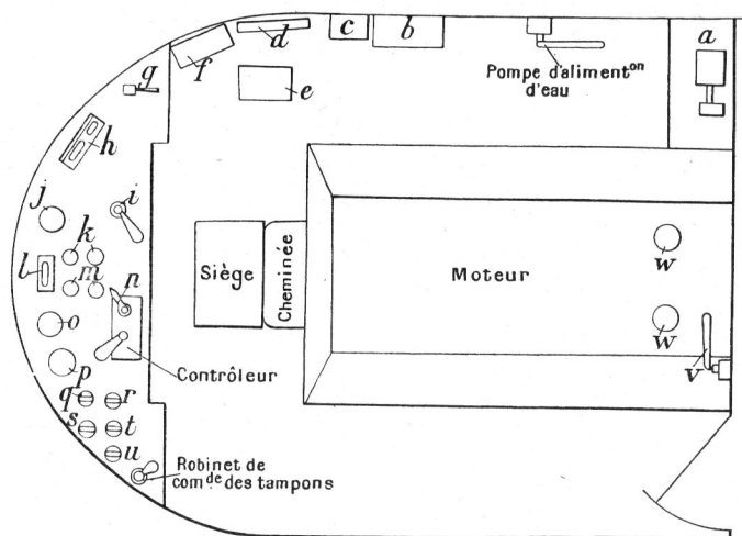
Plan schématique de la cabine de conduite.
