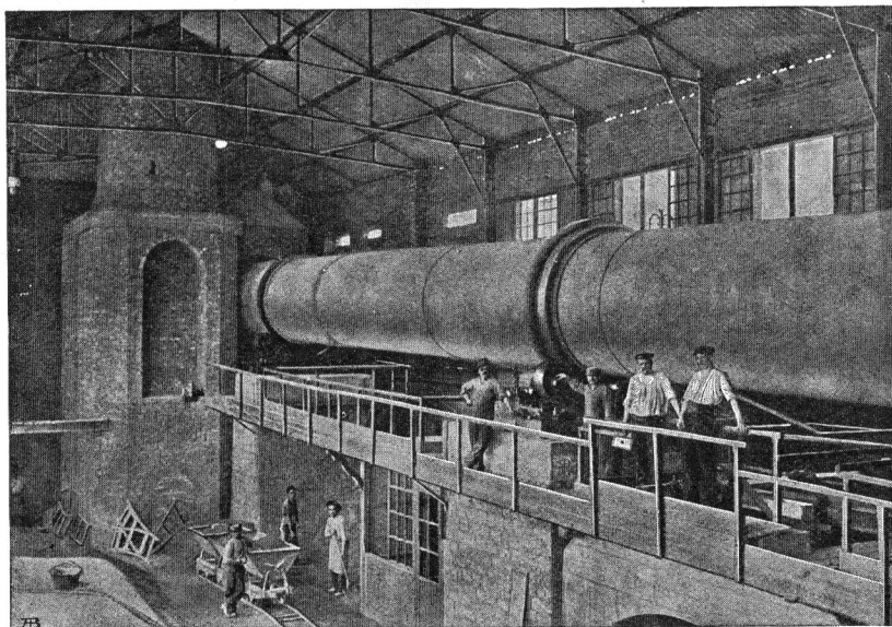
Four rotatif pour la cuisson du ciment.
