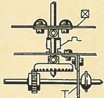
No. 97a Schnitt durch das Drehgestell Sezione del cavalletto di rotazione Section du chevalet giratoire Tväransnitt av vridstället.
