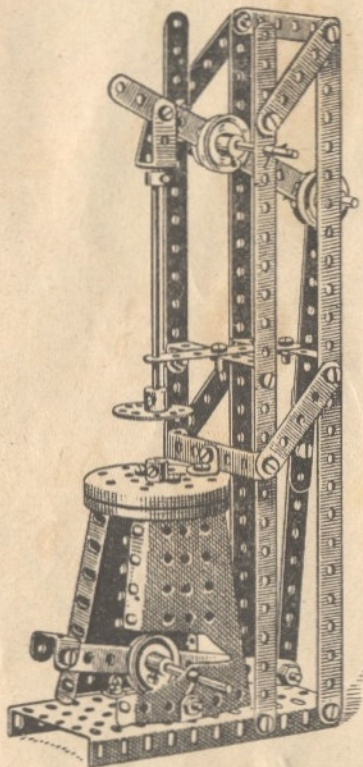
Fußtrittpresse
