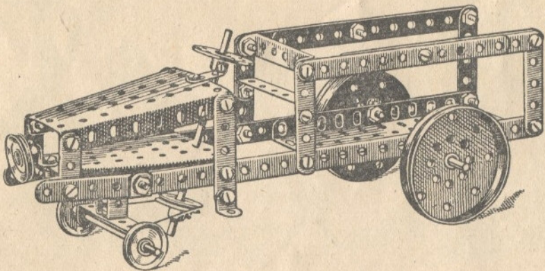
Kraftwagen
