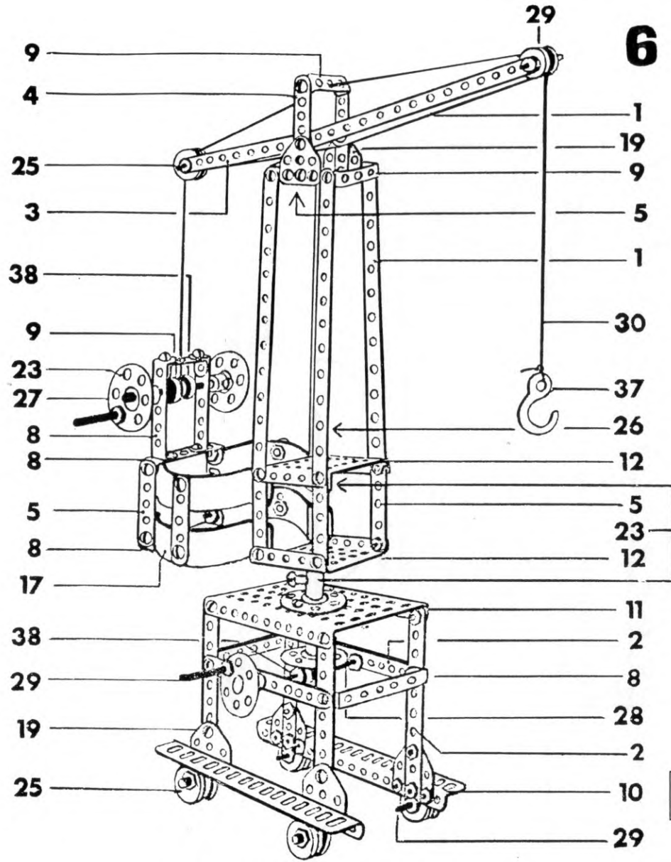
КРАН ПОДЪЕМНЫЙ
