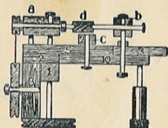
Drehbank, Längsschnitt
