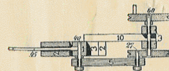
Dampfmaschine, Horizontalschnitt
