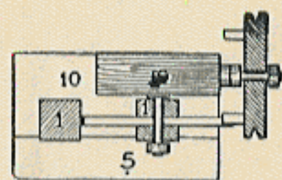
Nähmaschine Horizontalschnitt
