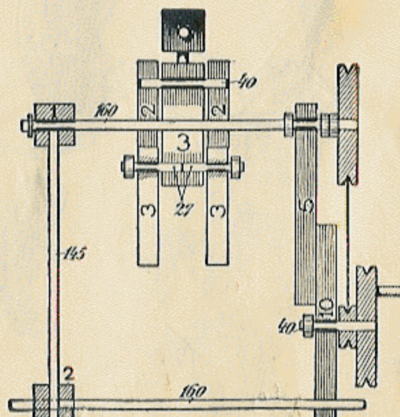
Reckturner, Querschnitt
