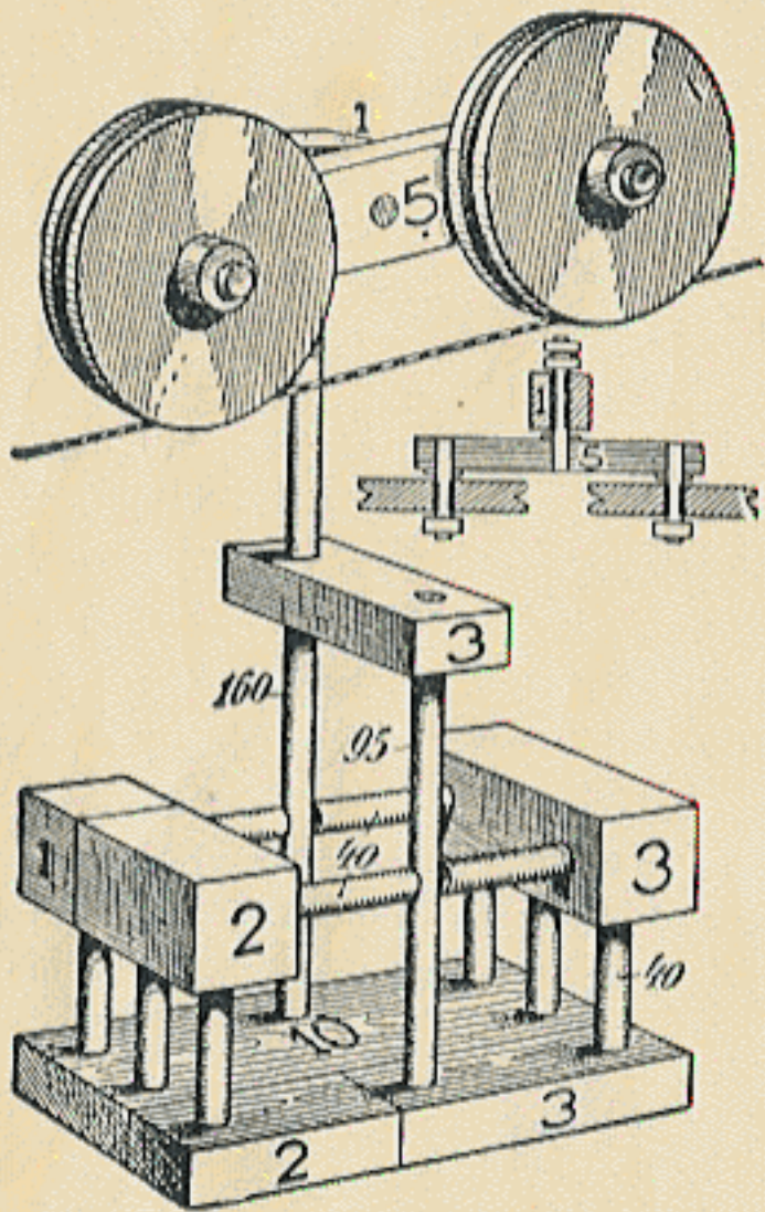
Hängeseilbahn
